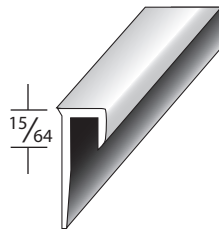
A-604H* 1/8" MAT'L MFA
