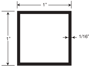
DIE 2724*
