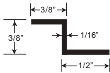
DIE 1447*
